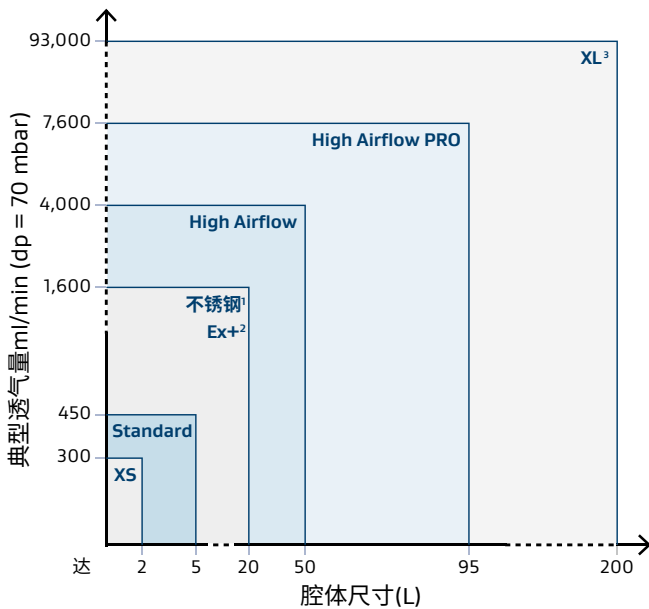
GORE® PolyVent螺纹系列产品组合
